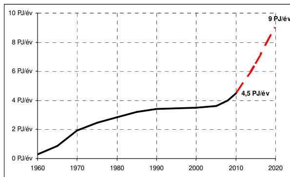
2. ábra A geotermia tervezett fejlődése 2020-ig
